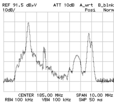
Abb. 1: Analoges TV-Signal
