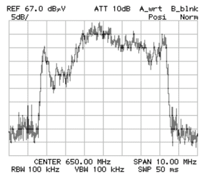
Abb. 3: DVB-T-Signal bei Mehrwegeempfang
