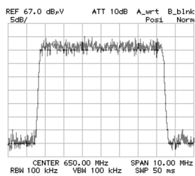
Abb. 2: DVB-T- Signal (ideal)
